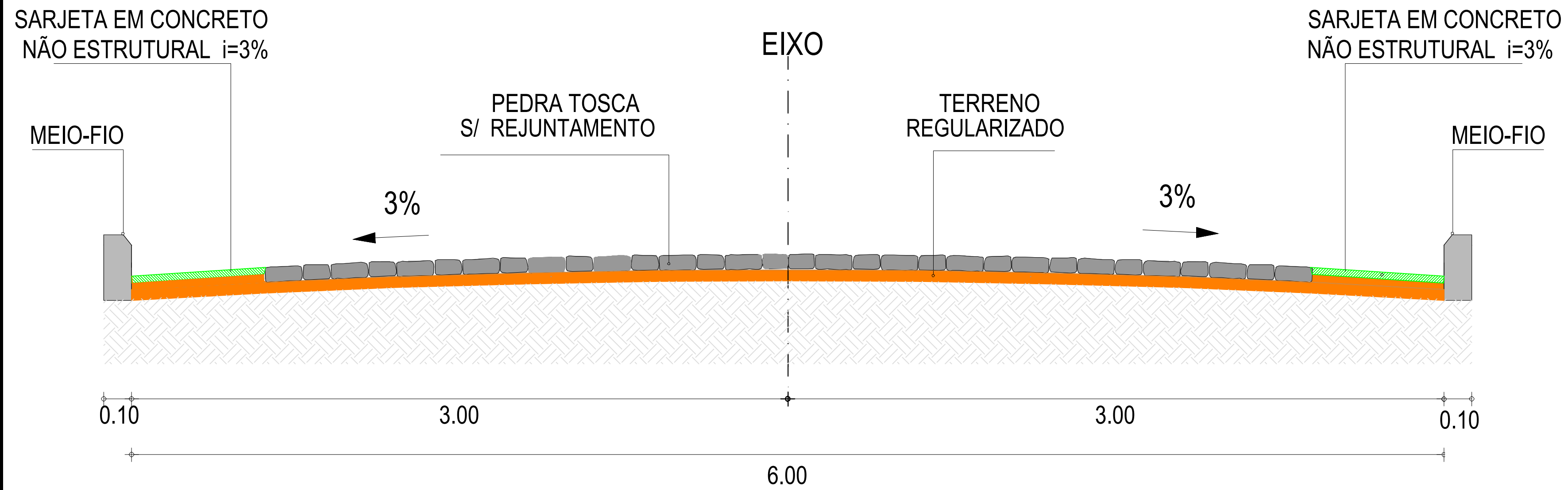
01 SEÇÃO TIPO PAVIMENTO ESCALA — 1 : SEM ESCALA
